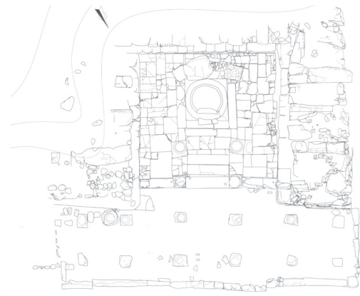
미륵대원지 보호석실 평면도
